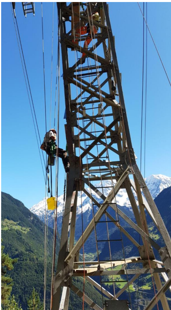
Masten 1; Sanierung 2017
